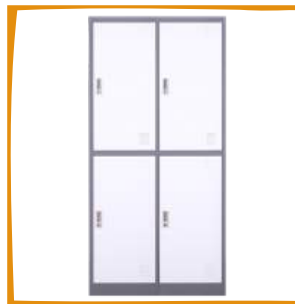
DNG-04 H1800*W900*D450
